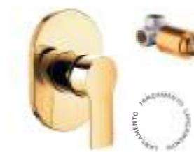
Ref. KR72670 Misturador monocomando para chuveiro. Base com cartucho de 40mm. Entrada de 3/4". Acabamento dourado [40838]. Acompanha base.
