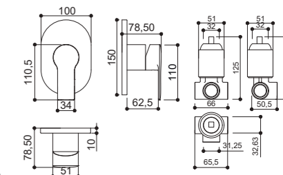
Ref. KR82670 Misturador monocomando para chuveiro. Base com cartucho de 40mm. Entrada de 3/4". Acabamento rose gold [40837]. Acompanha base.
