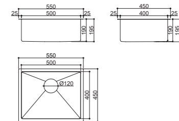
Ref. CUB2004 Acabamento dourado escovado [41026].
