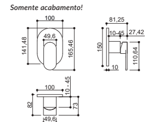
Ponteira de metal. Cartucho ø45mm
